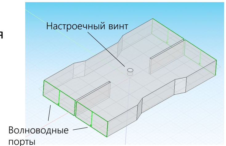
Модель ответвителя в ГАММА
